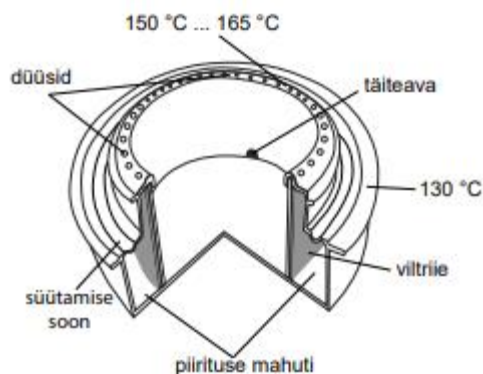
Pilt 1. Piirituspõleti läbilõige
